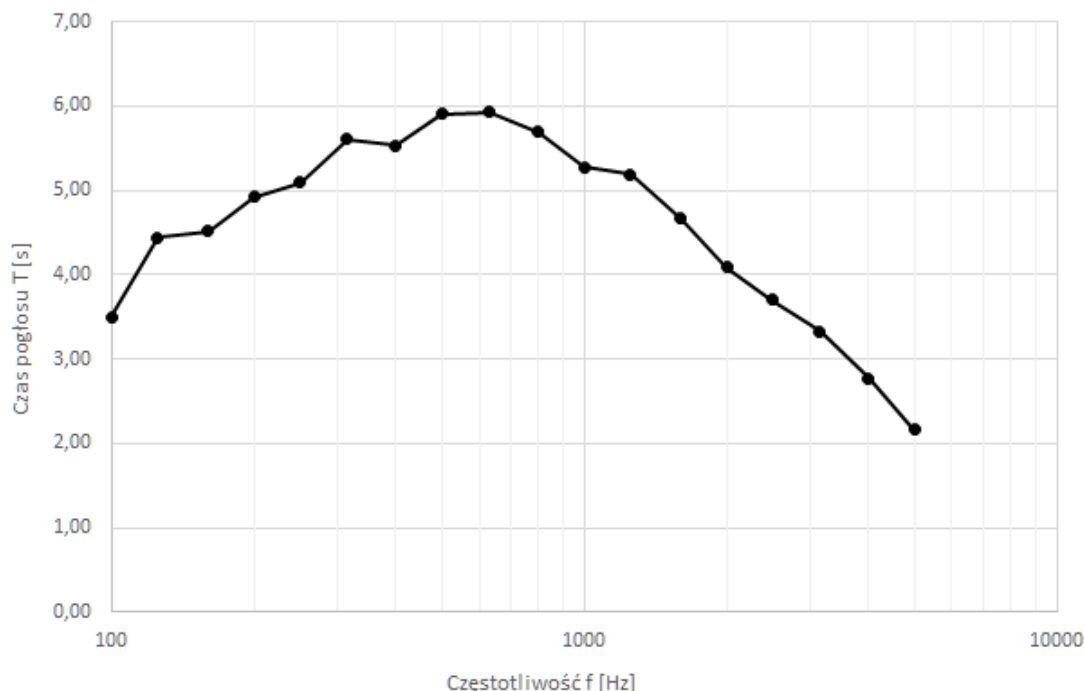
Wykres 3.1. Zmierzony czas pogłosu T_{20\text{śrt}} w funkcji częstotliwości
